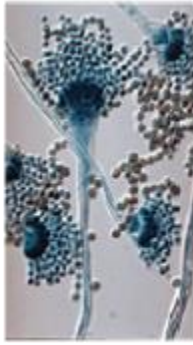
Aspergillus
