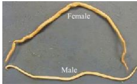
Ascaris
